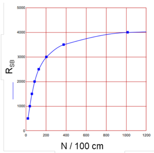
Figure 4. Variation de la capacité portante R_{SB} en fonction du nombre de coups
