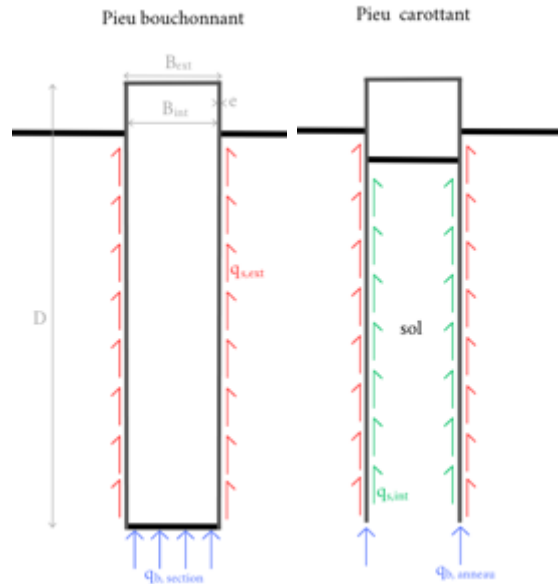
Figure 2. Termes de pointe et de frottement pour un pieu bouchonnant (à gauche) et pour un pieu carottant (à droite)
