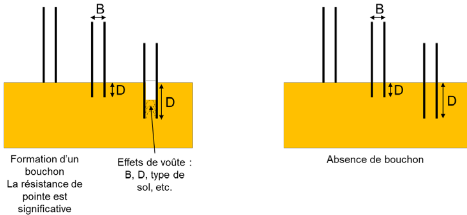
Figure 1. Comportement schématisé d'un pieu bouchonnant (à gauche) et carottant (à droite)
